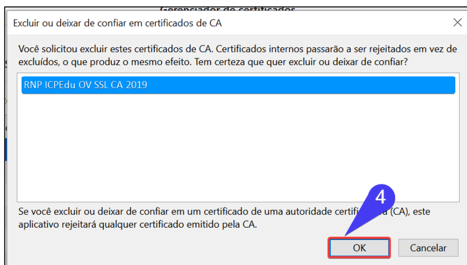
Figura 10 – Removendo certificado
