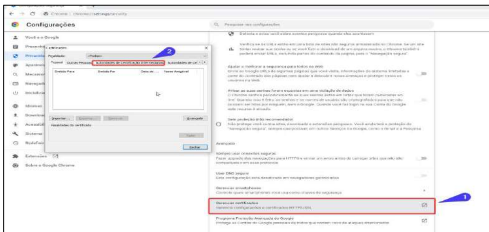
Figura 5 – Gerenciar certificados
