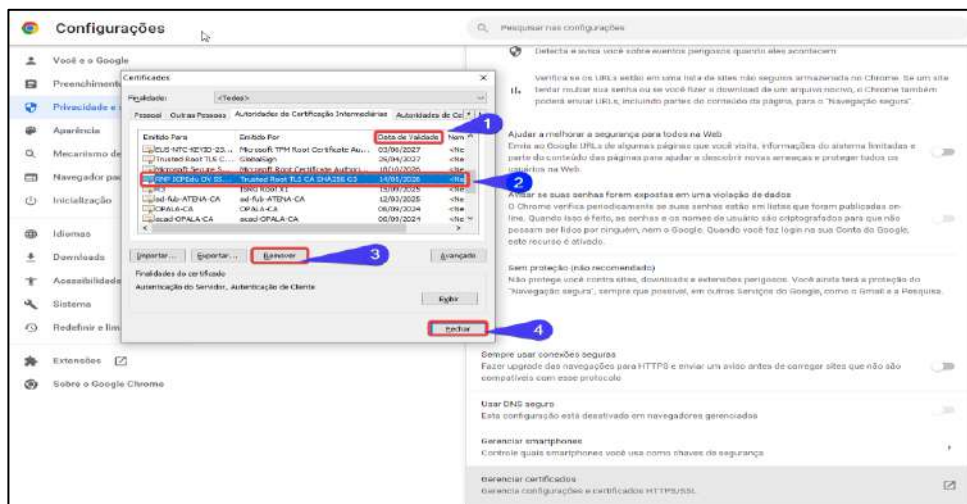
Figura 6 – Certificados
